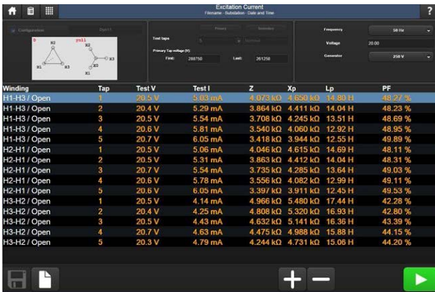
Ток возбуждения
