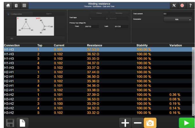
Сопротивление обмотки постоянному току
