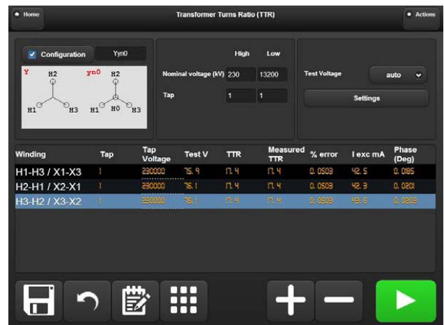
Коэффициент трансформации
